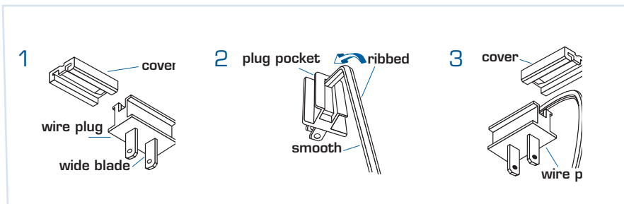
detachable plug
